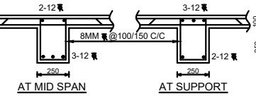
T-BEAM (B1)
