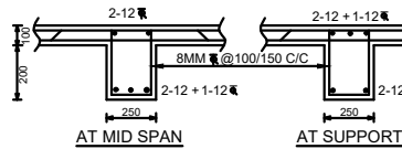
T-BEAM (B2)
