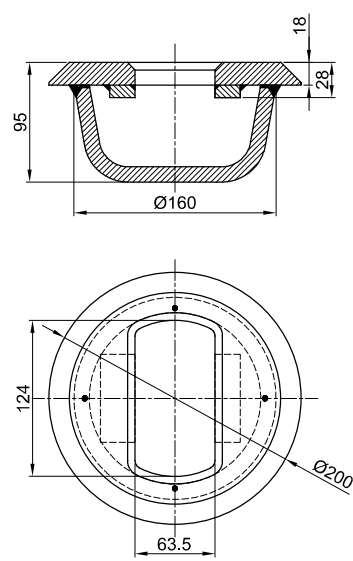
FLUSH DECK SOCKET : TYPE - A (Qty - 24 Nos.)
