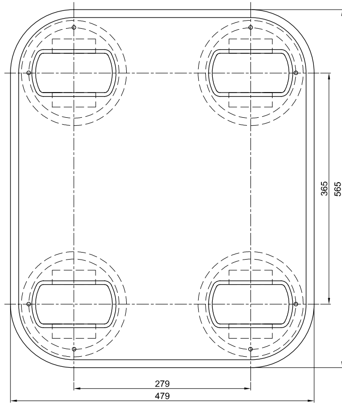
FLUSH DECK SOCKET : TYPE - D (Qty - 22 Nos.)
